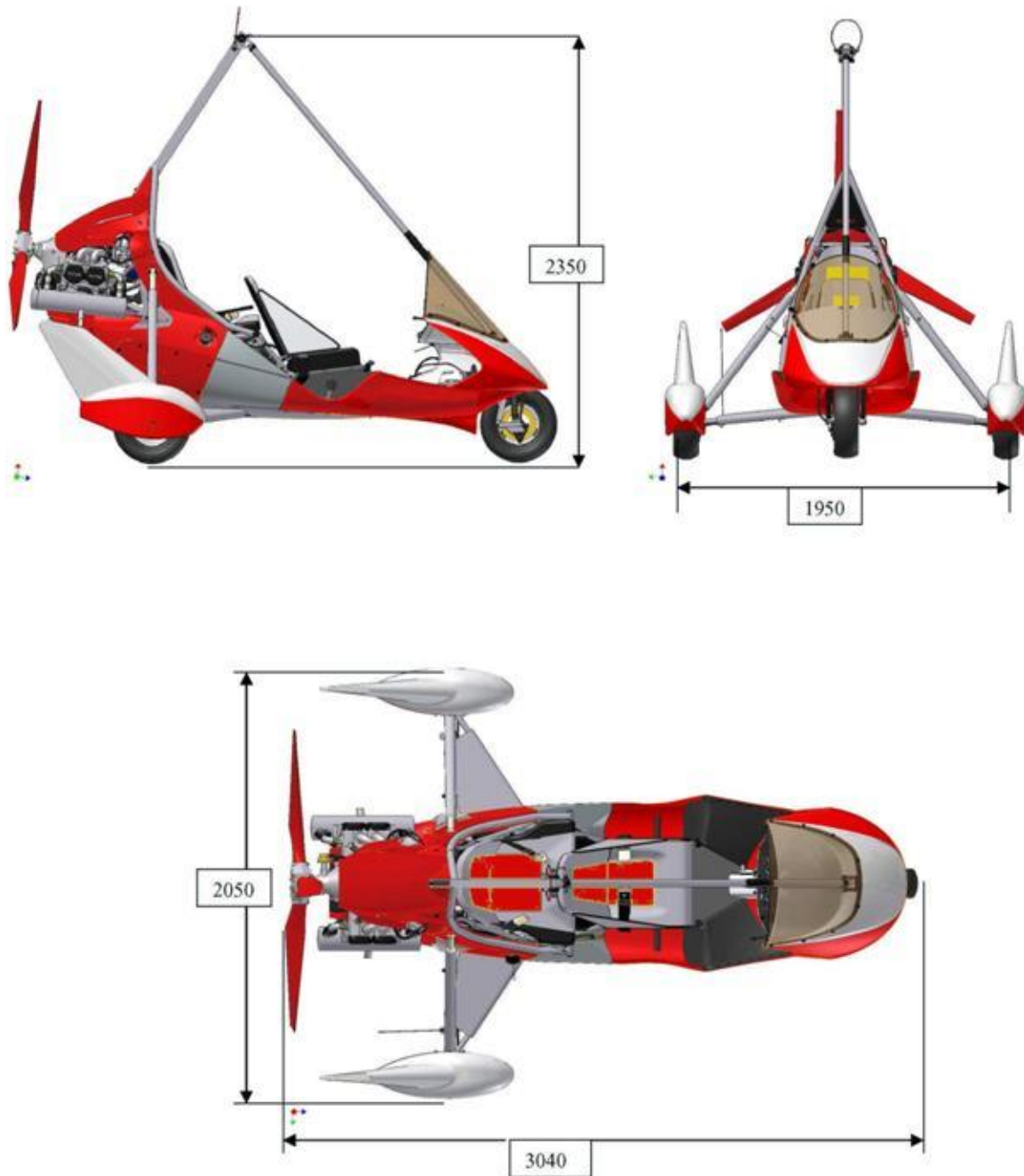
Figure 3-1 : Tanarg 912 - 3 Vues
