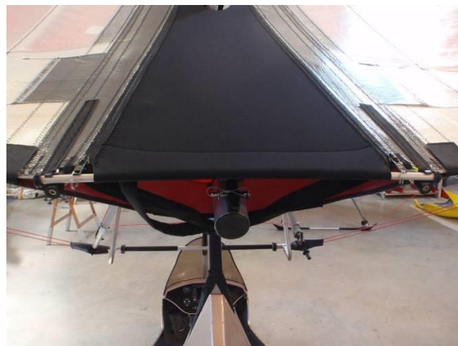
Figure 5-4 : Latte centrale de Bord de Fuite
